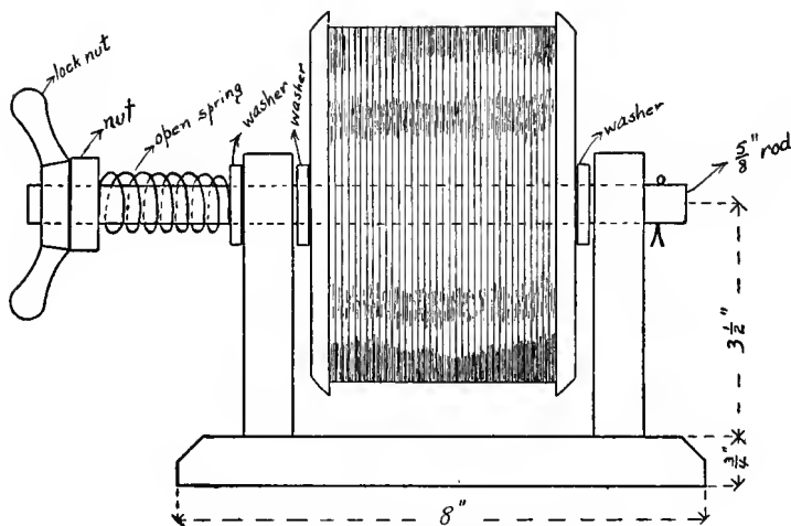
FIG. 4. — WIRE-SPOOL HOLDER.
