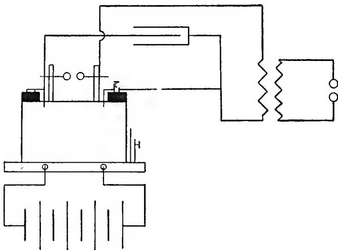
FIG. 49. — WIRING DIAGRAM.
