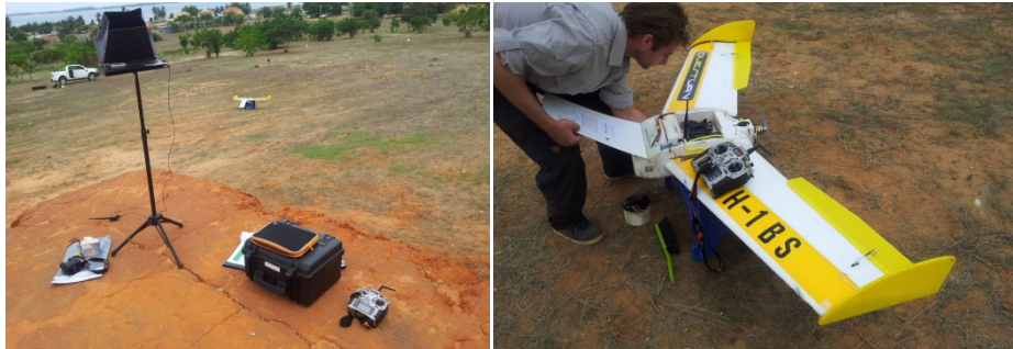
Sistema de Levantamento aéro-topográfico por “drone”
