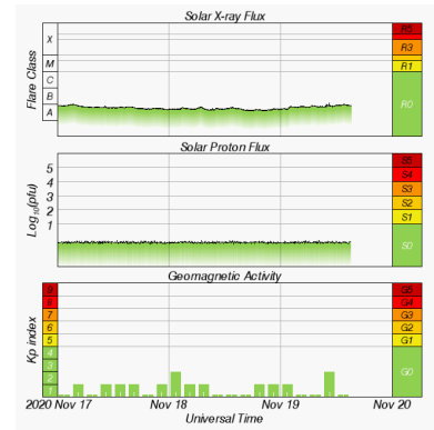
SWPC / NOAA
